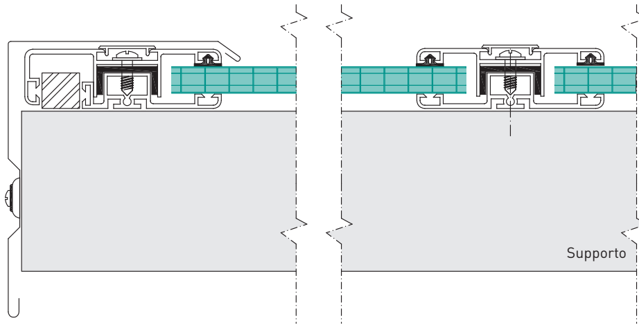
SCHEMA [ A ] Profilo di testata in alluminio
